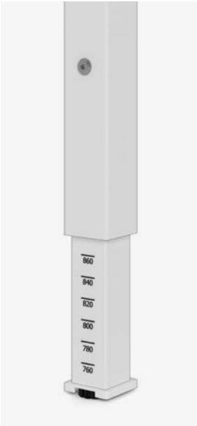
h 62 ÷ 86 cm Regolazione in altezza ogni 2 cm Height adjustment every 2 cm Réglage hauteur tous les 2 cm Höhenverstellung alle 2 cm Ajuste de altura cada 2 cm
