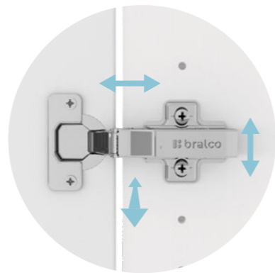
anta con cerniera regolabile montata door with levelling hinge porte avec charnière réglable montée Tür mit montiertem einstellbarem Scharnier deur met gemonteerde, verstelbaar scharnier puerta con bisagra regulable montada
