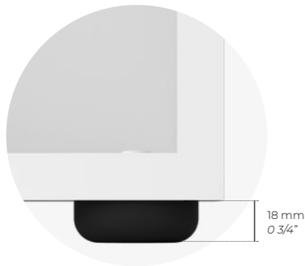
pedino livellatore levelling foot vérin de compensation Niveausgleichsfuss stelpoot pie nivelador
