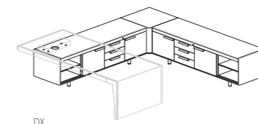
DX CX2922 (DX) L256,4 P256,4 H61,6 CX2921 (SX) L256,4 P256,4 H61,6
