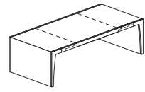
CX0519W L188 P91,7 H75 CX0521W L210 P101,7 H75 CX0523W L234 P101,7 H75
