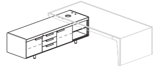
SX CX2906 (DX) L193,5 P57 H61,6 CX2905 (SX) L193,5 P57 H61,6
