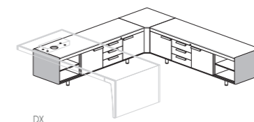
DX CX2932 (DX) L256,4 P256,4 H61,6 CX2931 (SX) L256,4 P256,4 H61,6
